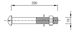
취부볼트 SCALE: NONE
