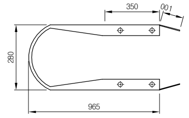
라운드레일 SCALE: NONE
