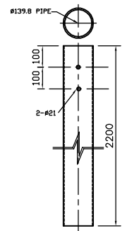
PIPE POST 상세도
