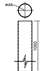
지주보강재상세도
