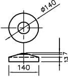
지주캡 상세도
