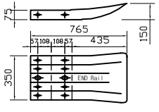
단부레일 상세도
