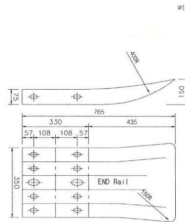
편면도
