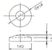
지주캡 상세도
