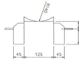
편면도
