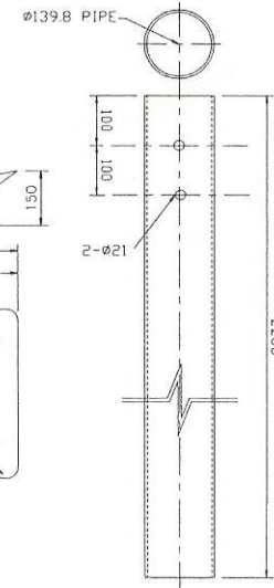
PIPE POST 상세도
