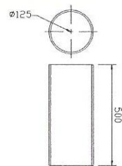
지주보강재상세도
