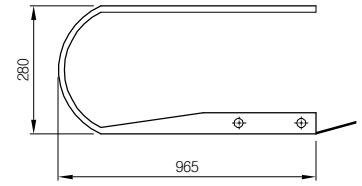
라운드레일 SCALE: NONE
