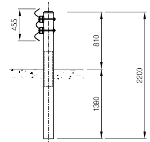
SIDE ELEVATION SCALE: NONE
